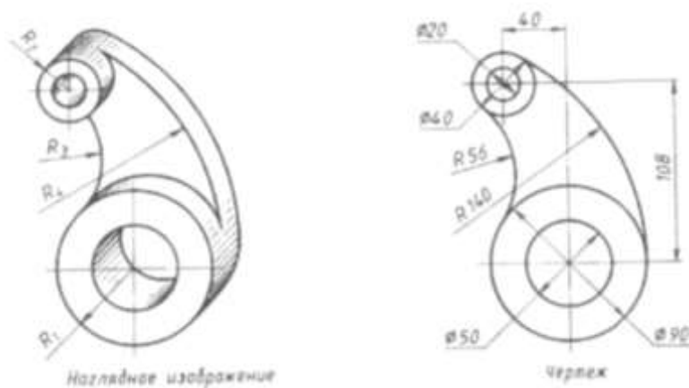
Графическая работа №4 «АксонOMETрическая проекция детали»
